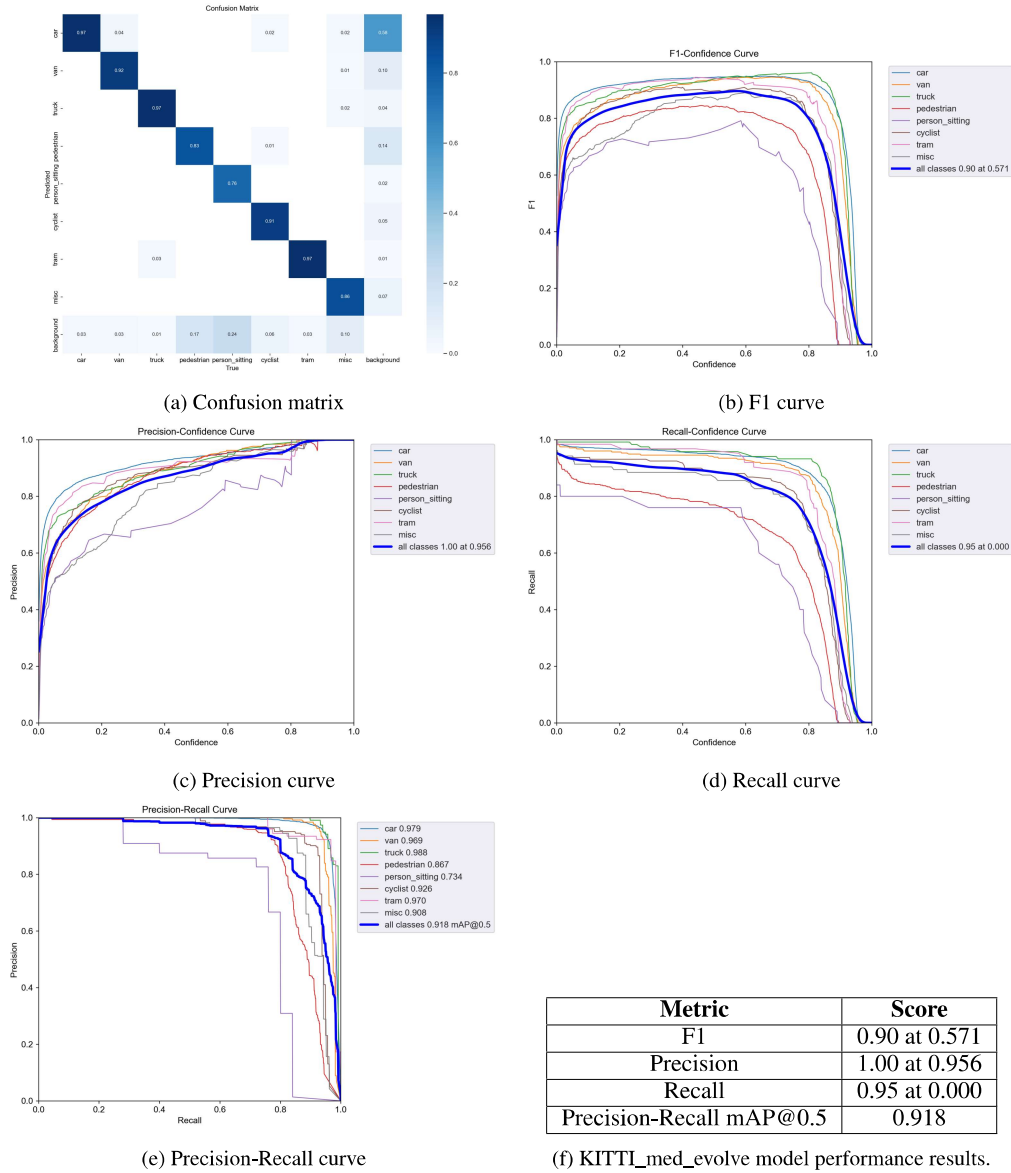
Figure 15: KITTI_med_evolve result metrics
